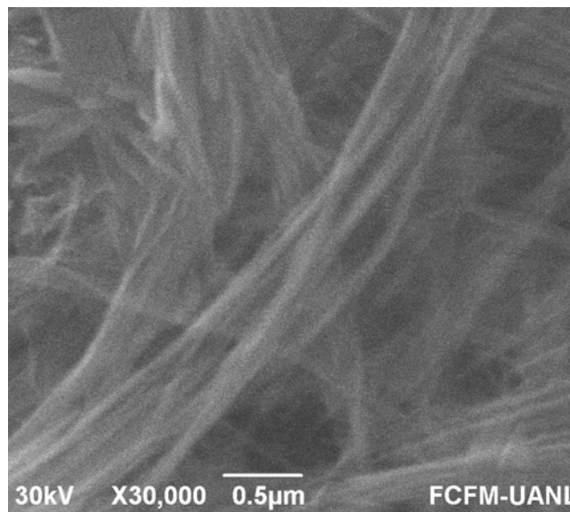
Figura 4. Imágenes SEM de nano alambres de \text{Cu}(\text{OH})_2 .
