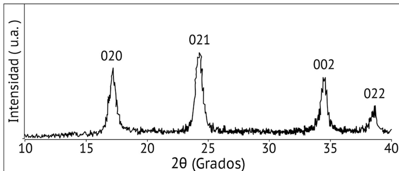
Figura 3. Patrón XRD de nano alambres de \text{Cu}(\text{OH})_2 .
