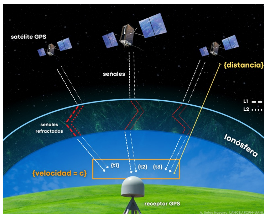
Figura 2. Diagrama del Sistema de Posicionamiento Global (GPS) y su interacción con la ionósfera terrestre. Las líneas punteadas indican las señales L1 y L2, enviadas por los satélites (fuente: elaboración propia).
